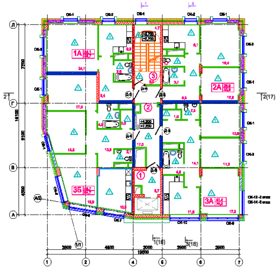
Схема расположения квартиры на этаже корпуса № 5
