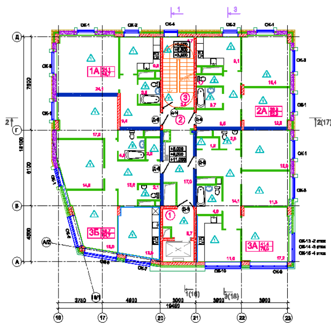
Схема расположения квартиры на этаже корпуса № 6
